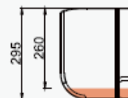
Side View 側面圖
